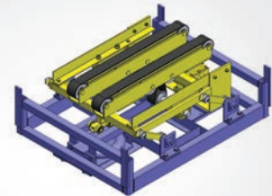
Neukonstruktion Eckumsetzer für Fa. Radsysteme GmbH
